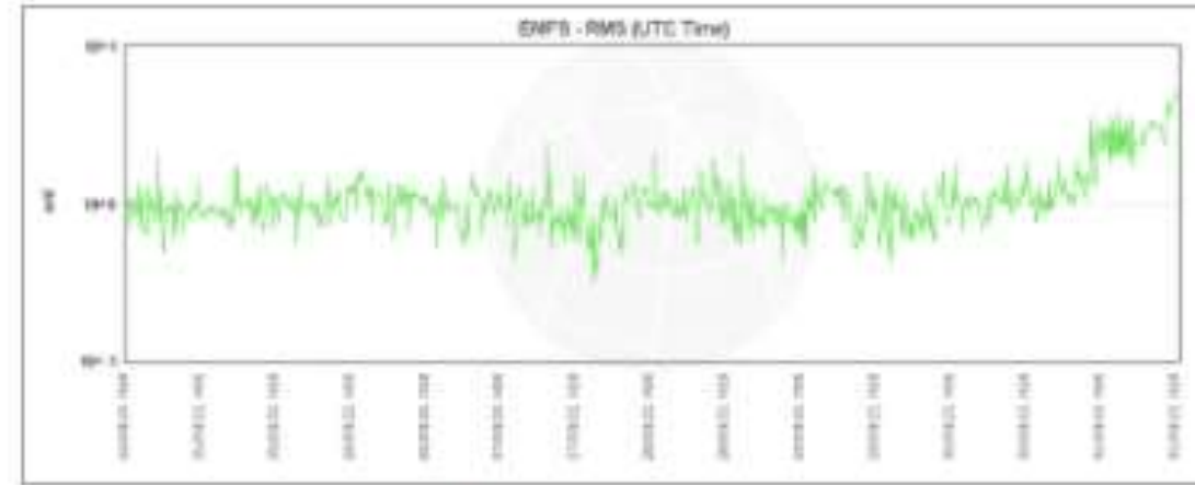
Rising tremor signal (image: INGV Catania)
